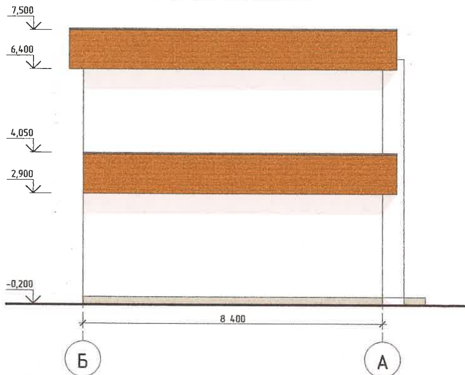
Фасад в осях Б-А
