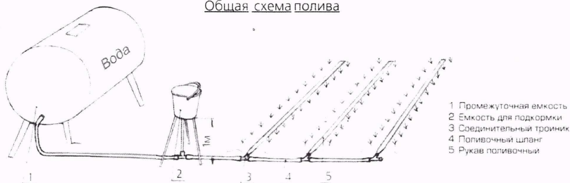
Общая схема полива
