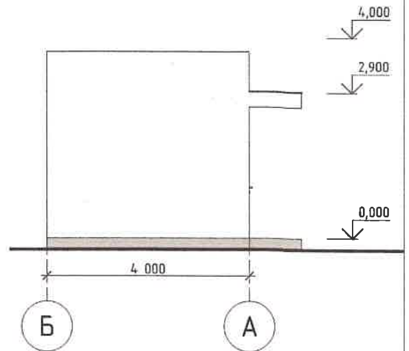
Фасад в осях Б-А
